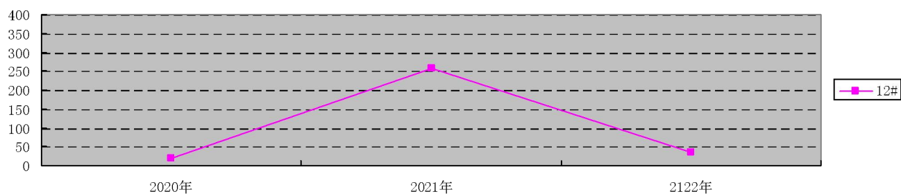
图 5.3-2 氯化物超 V 类点位浓度趋势图 (V 类 > 350mg/L)
