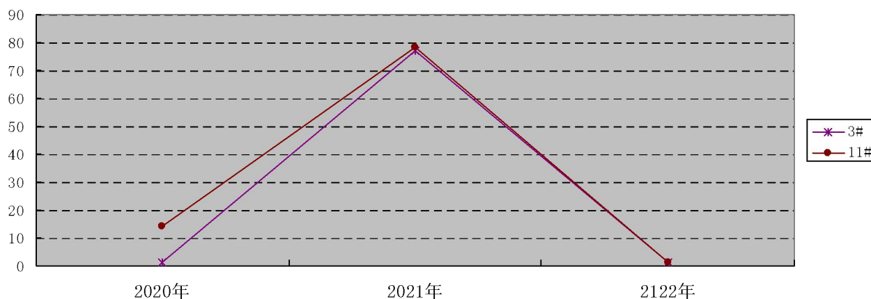
图 5.3-8 1,2-二氯乙烷超V类点位浓度趋势图（V类>ug/L）
