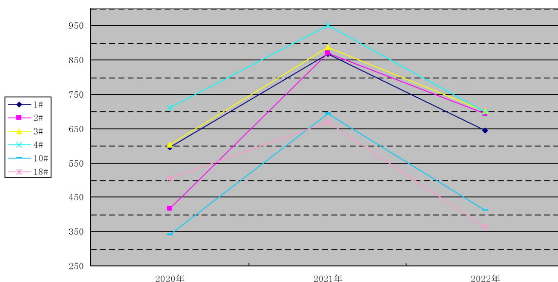
图 5.3-1 总硬度超V类点位浓度趋势图（V类>650mg/L）
