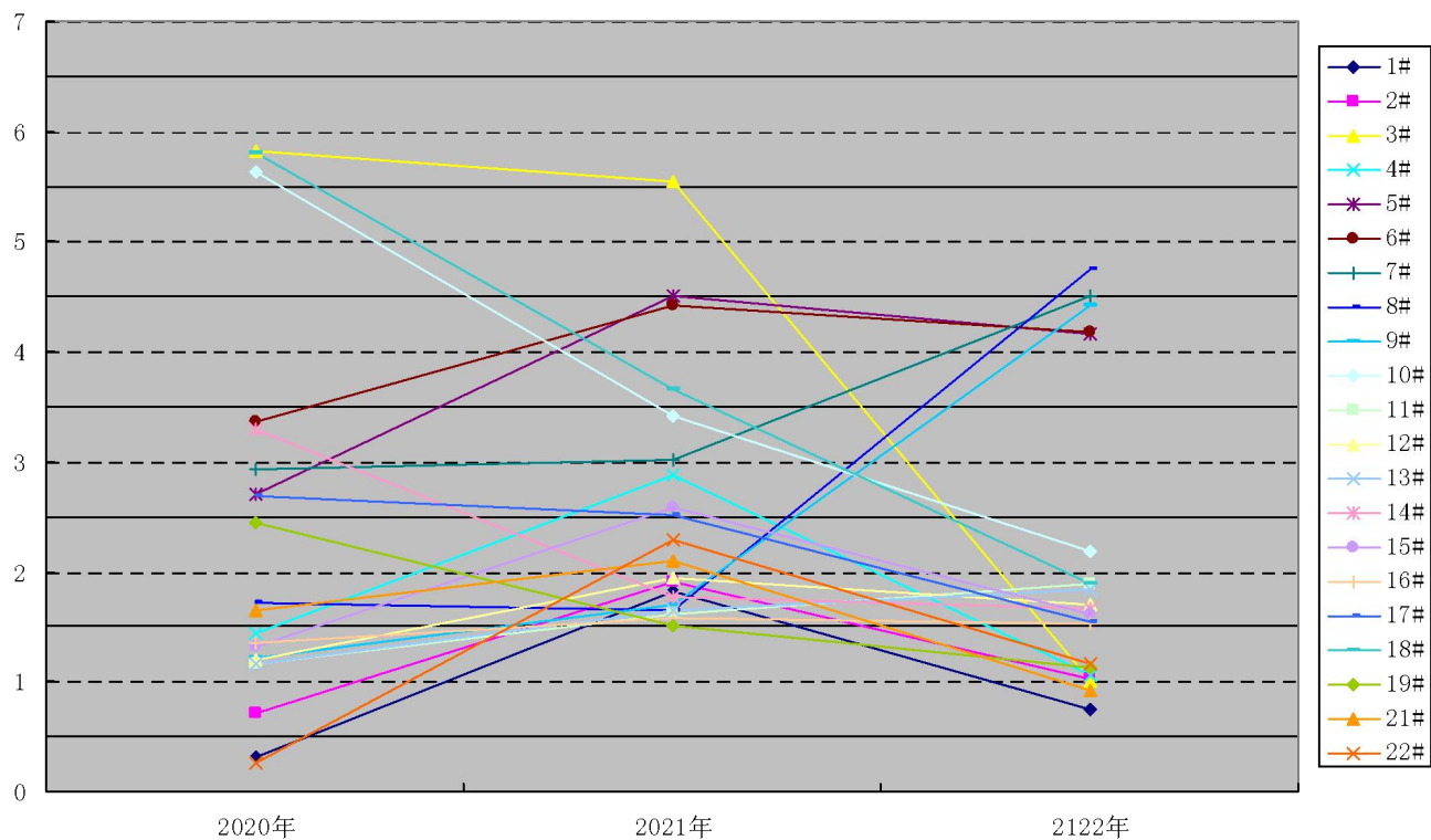
图 5.3-6 氨氮超V类点位浓度趋势图（V类>1.5mg/L）
