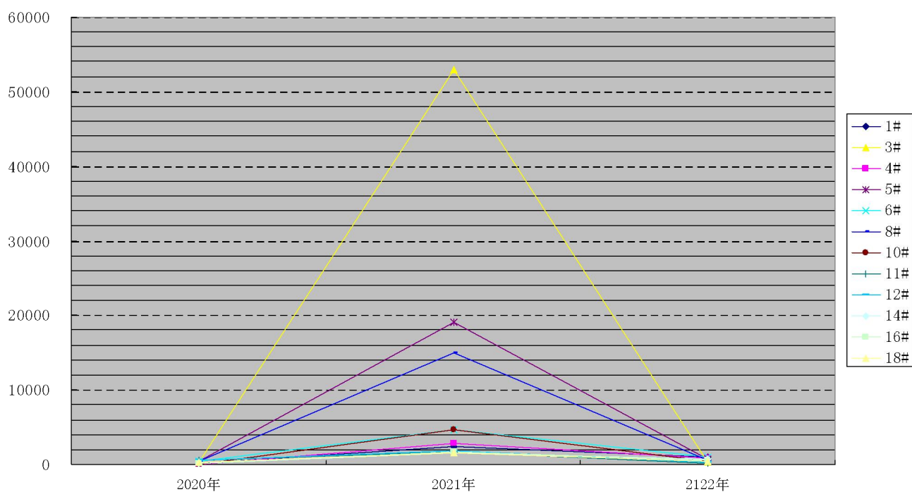
图 5.3-7 细菌总数超V类点位浓度趋势图（V类>1000CFU/mL）
