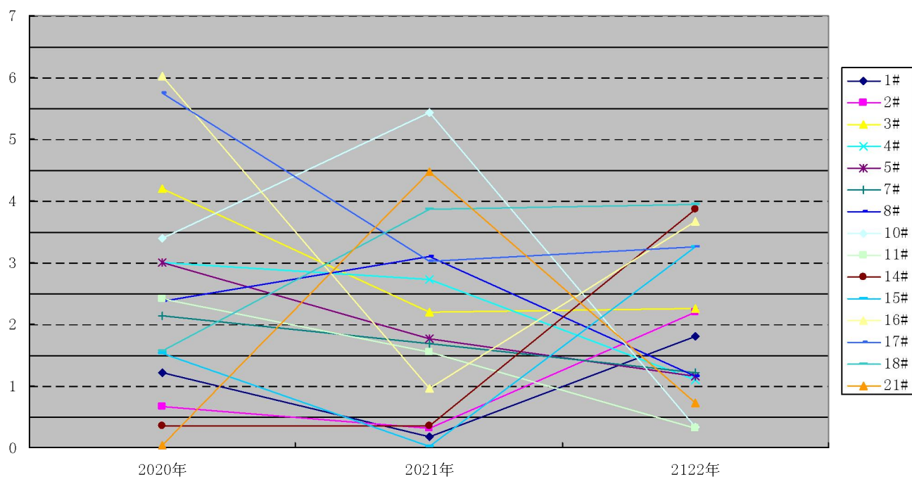
图 5.3-4 锰超V类点位浓度趋势图（V类>1.5mg/L）
