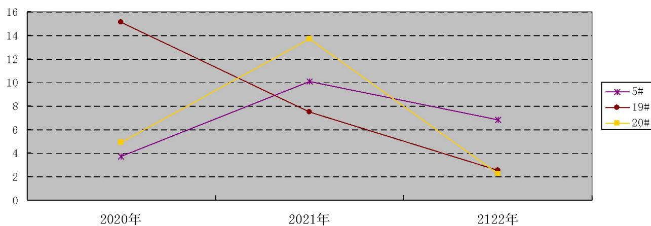
图 5.3-5 耗氧量超V类点位浓度趋势图（V类>10.0mg/L）
