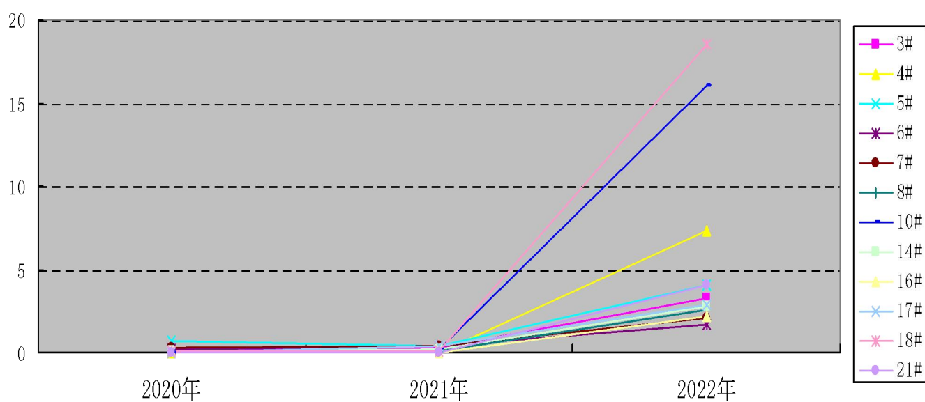
图 5.3-3 铁超 V 类点位浓度趋势图 (V 类 > 2.0mg/L)
