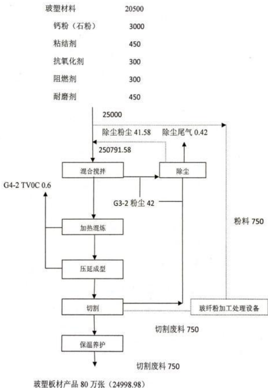
图 4.1-3 板材生产工艺流程及产污环节
