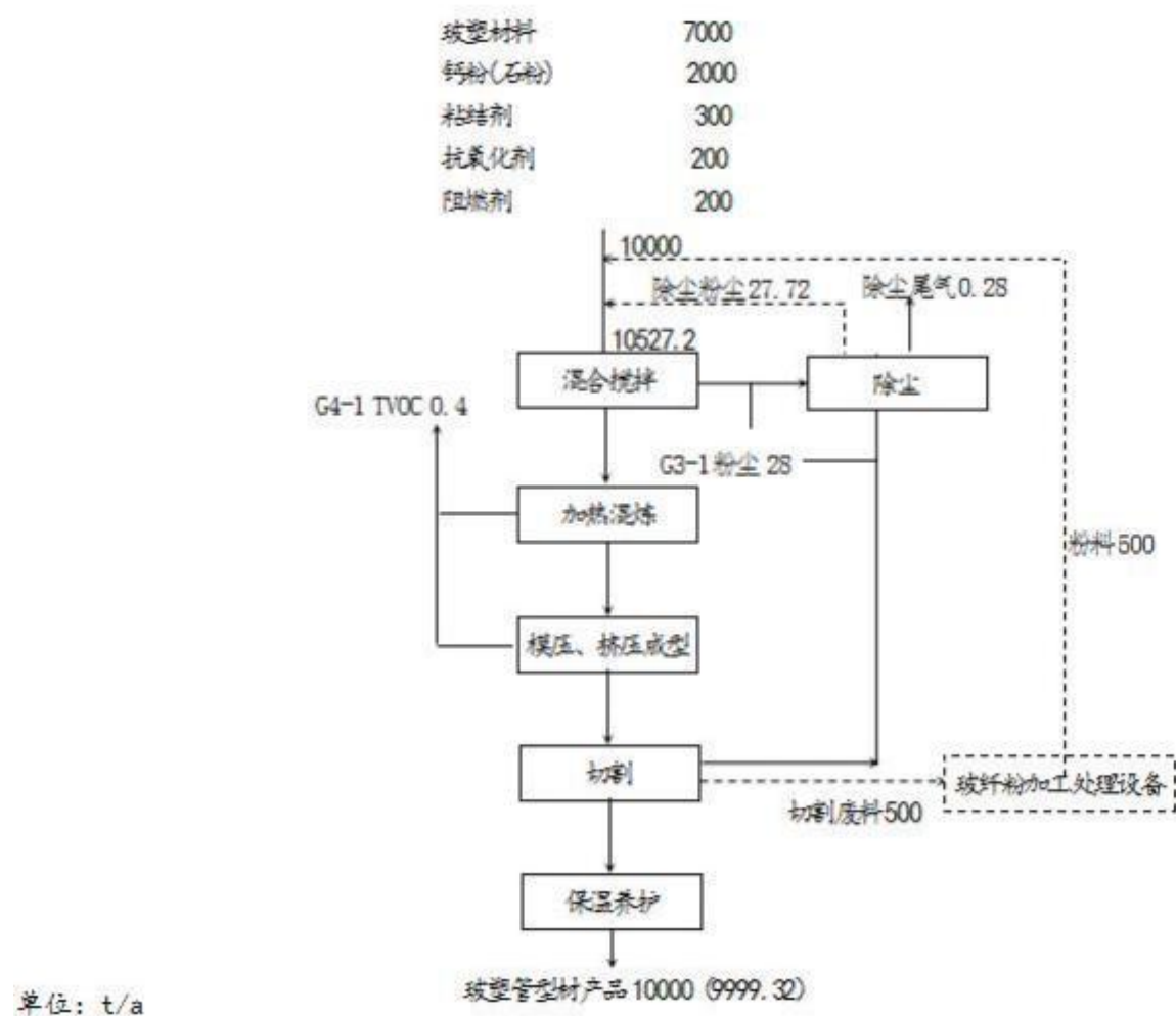
图 4.1-2 玻塑管型材生产工艺流程及产污环节
