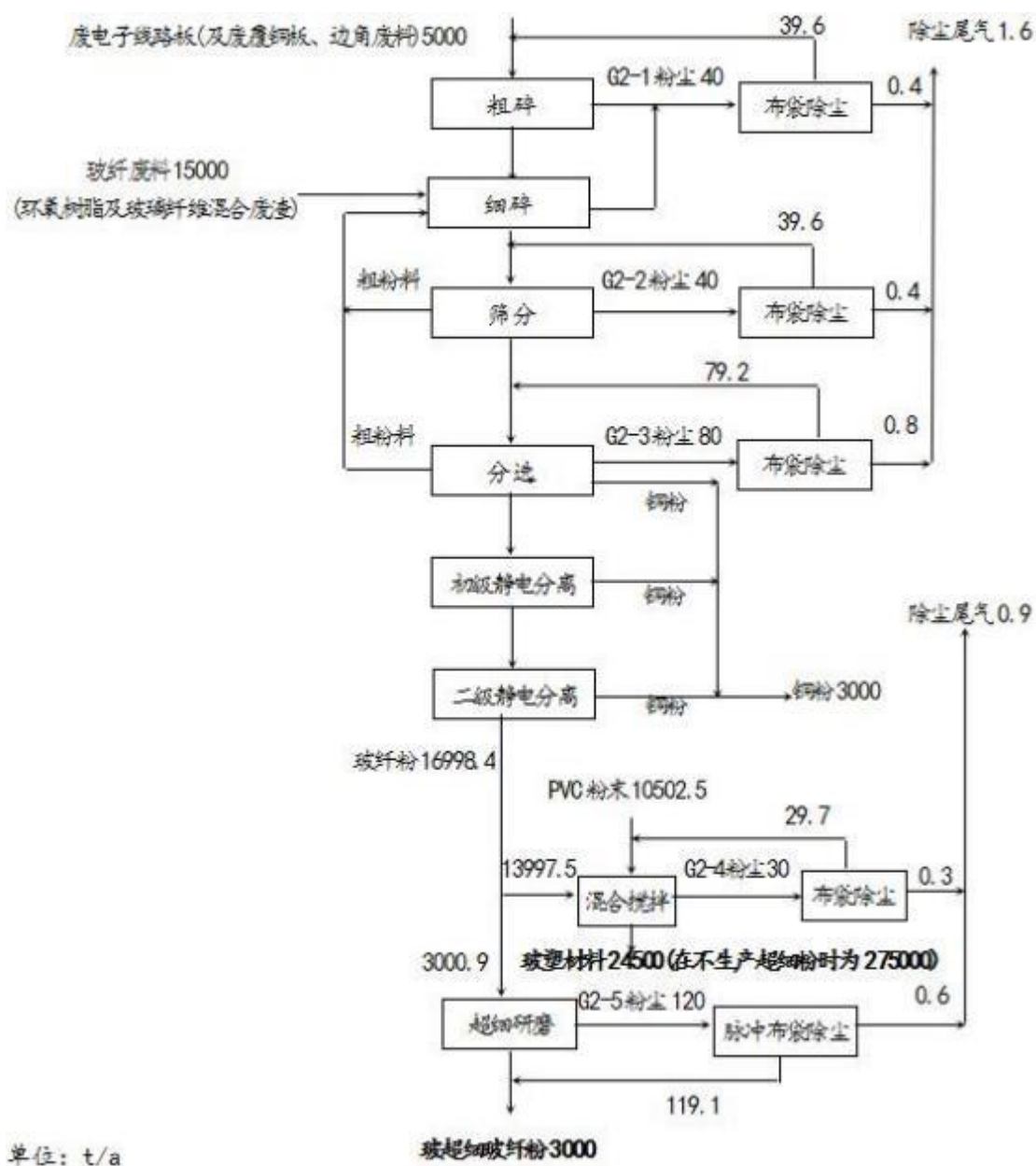
图 4.1-1 废旧线路板（及废覆铜板、边角废料）、树脂玻纤废料加工处理工艺流程及产污环节
